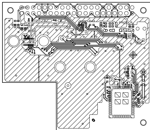
部品面パターン
