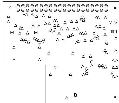
穴図 ( 部品面視 )
