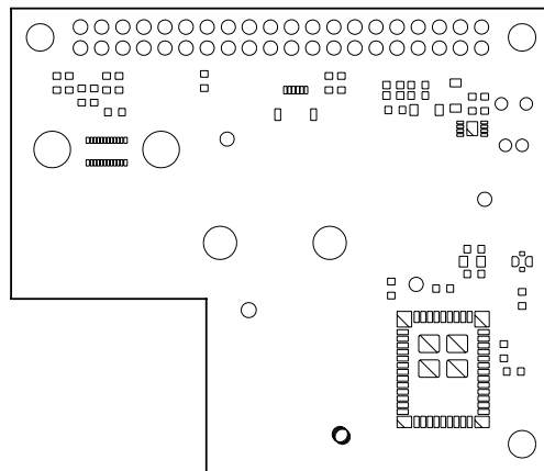
部品面レジスト
