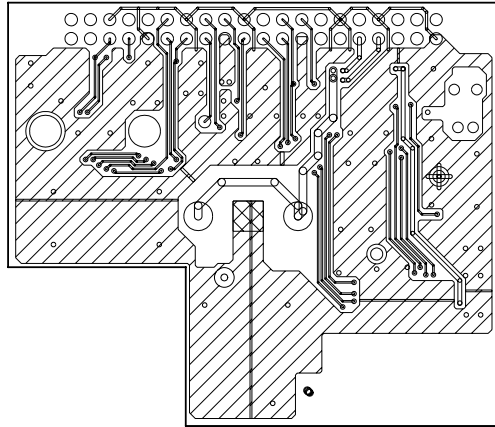
半田面へのルーティング
