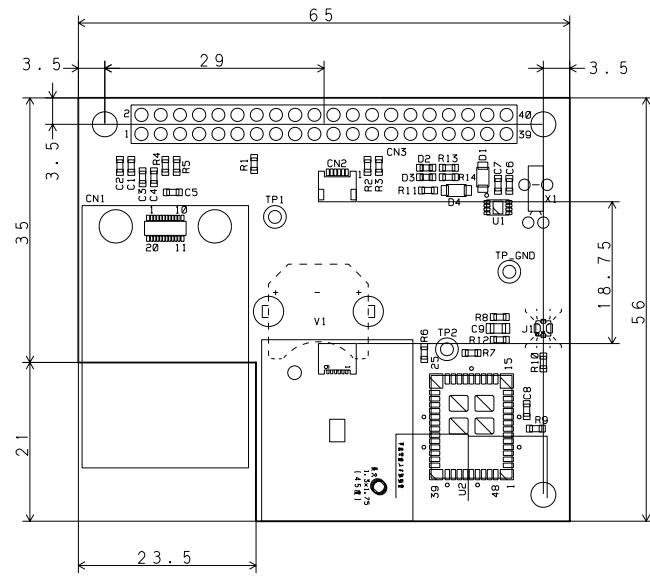
部品面レジスト 集積図 (部品面)
